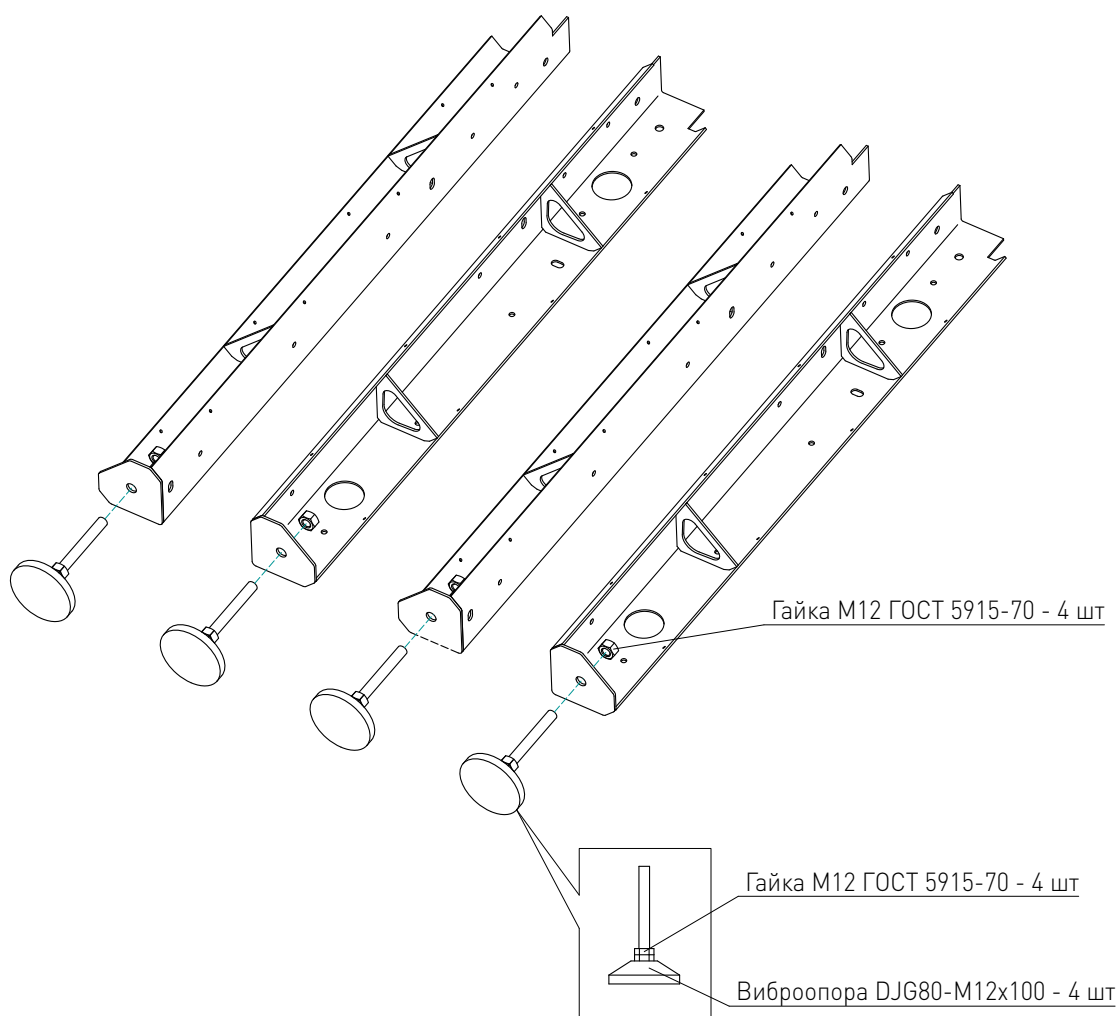
Рисунок 3 — Сборка опор.
