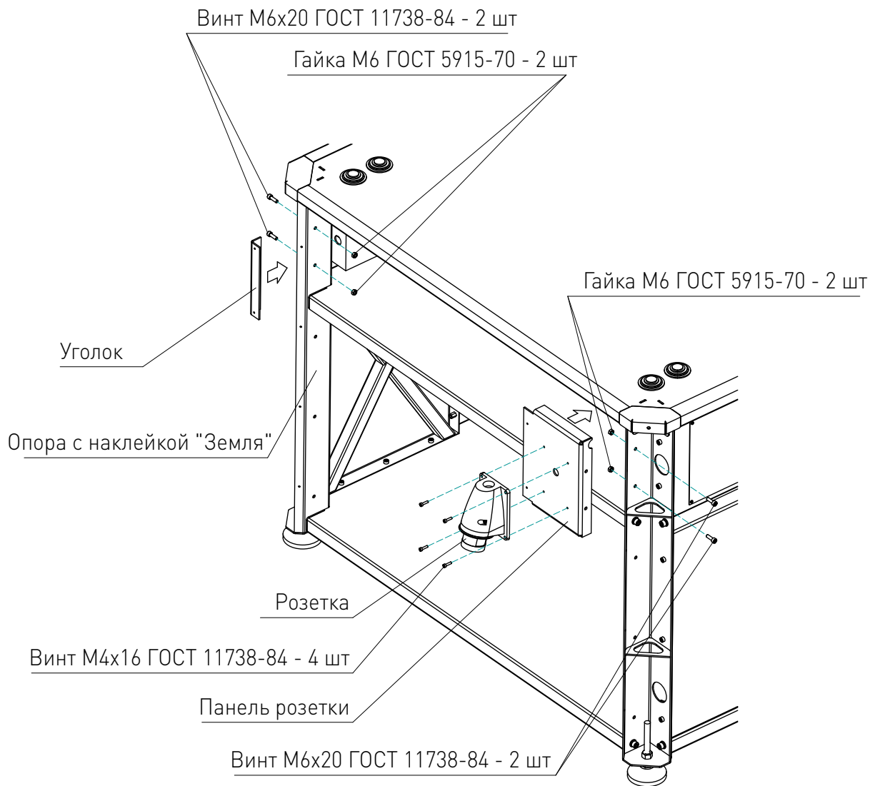
Рисунок 9 — Установка розетки.
